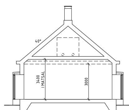
SEKTION
