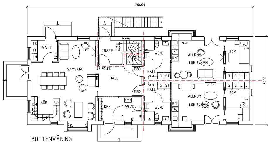
BOTTENVÅNING
