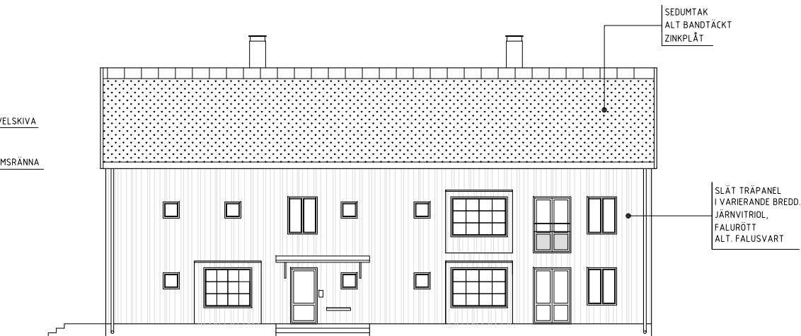
FASAD FRAMSIDA
