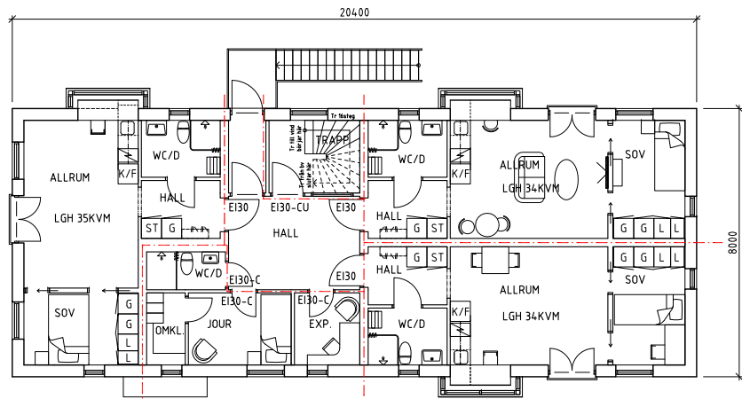
VÅN 1TR
