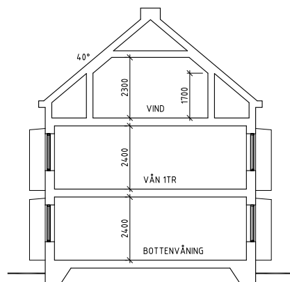
SEKTION
